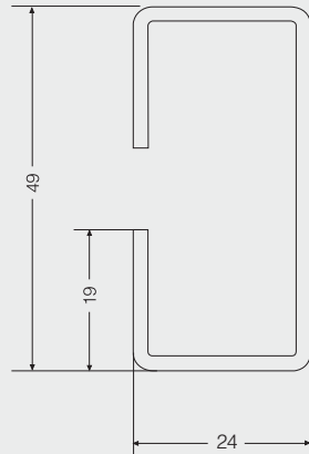
YP Yatay Profil Kesiti
