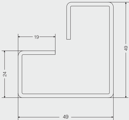
DP Dikey Profil Kesiti
